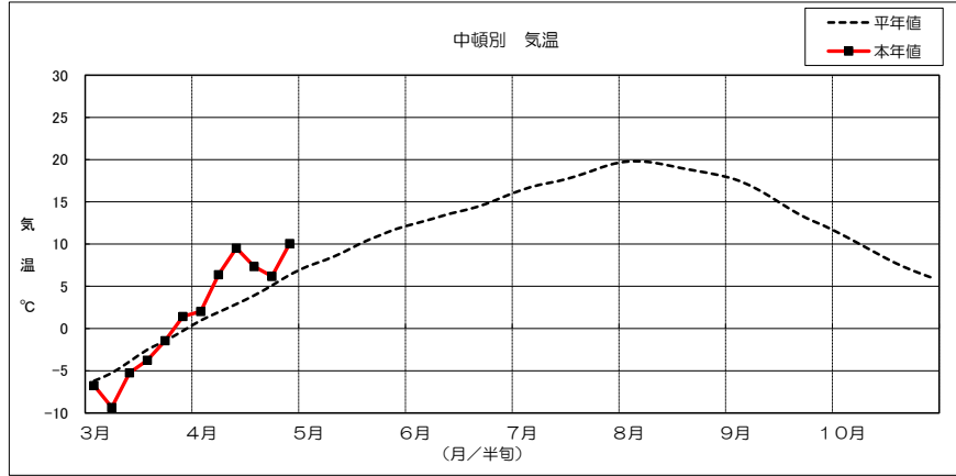
2024年気象経過図(中頓別アメダス)
