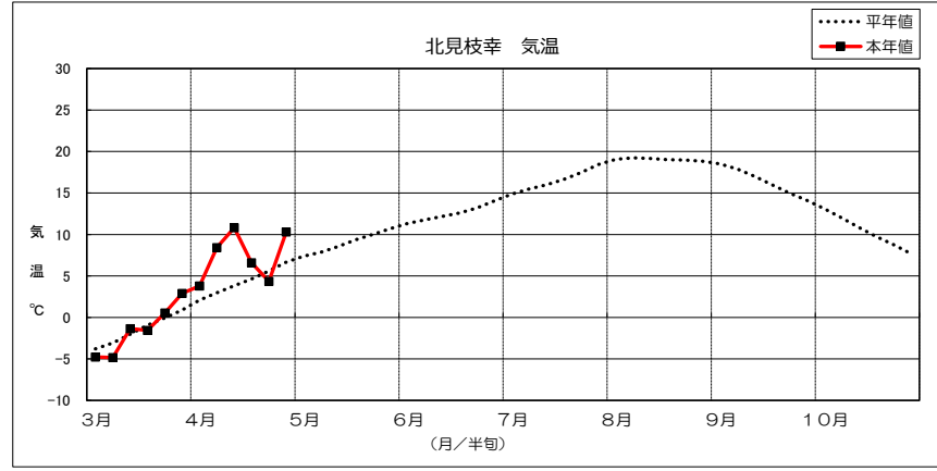
2024年気象経過図(北見枝幸アメダス)
