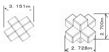
六脚ブロック A1.00型 (囲いブロック)
