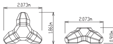
截頭シェイクブロックII型 (囲いブロック)
