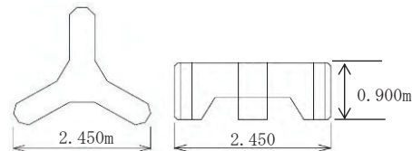
SGブロック 2.7t型 (囲いブロック)
