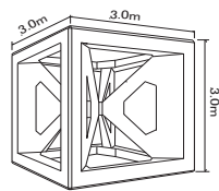
FP魚礁3.00型 (魚礁ブロック)
