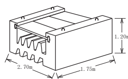
SKKブロック (増殖礁ブロック)
