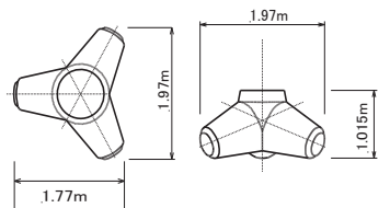
サイ頭テトラポッドS-25型 (囲いブロック)
