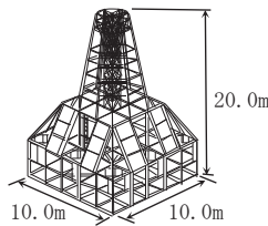
截頭シェイクブロックII型 (囲いブロック)
