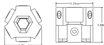
オクトム(2段積み) (ミズダコ産卵礁)
