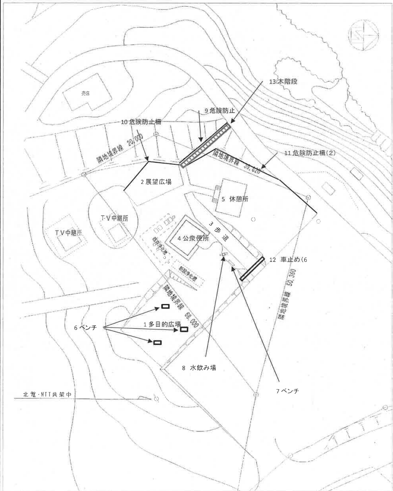
施設配置図(全体平面図)及び施設写真(全景)
